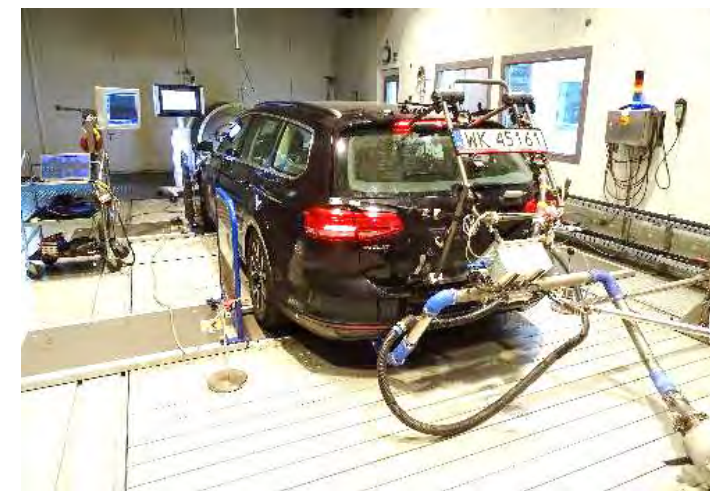
Weryfikacja instalacji PEMS na hamowni podwozia
